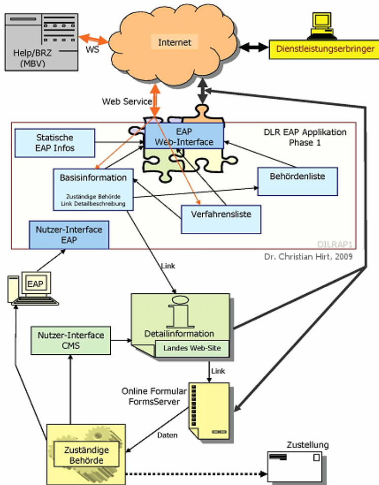
Übersicht Architektur DLR Umsetzung (Phase 1)
